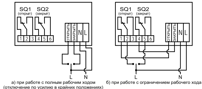
Рисунок 3 Схема подключения
