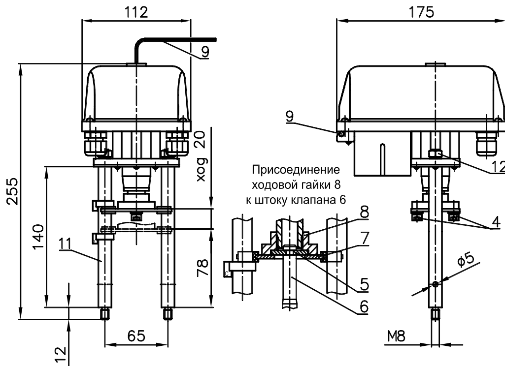
Рисунок 1 - ВЭП-115В
