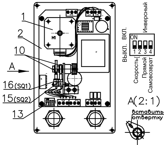
Рисунок 2 - ВЭП-118В (вид при снятой крышке)
