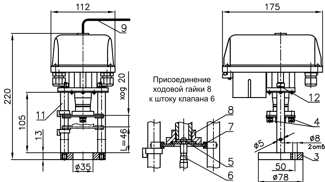
Рисунок 1 - ВЭП-118В
